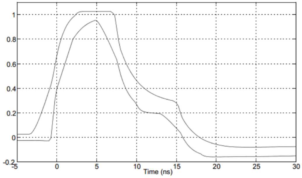
图 8-1 A、B、C、D 点模板
