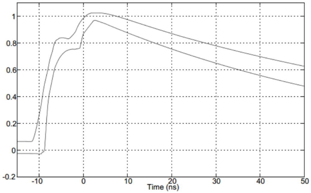
图 8-2 F、H 点模板
